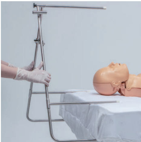
本体の設置は、縦方向、横方向から可能です。 脚部分は170mmまでのベッドマットを挟むことができます。
